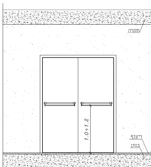
תרשים 14 : דלת עם מנעול בהלה
